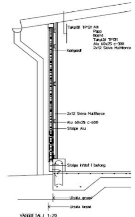
Väggdetalj
