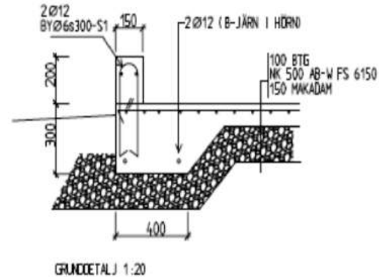
Grunddetalj
